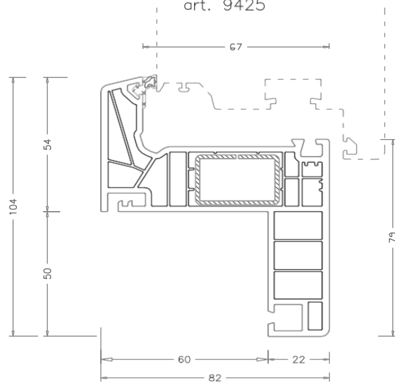
Telaio Z 50 mm art. 9425
